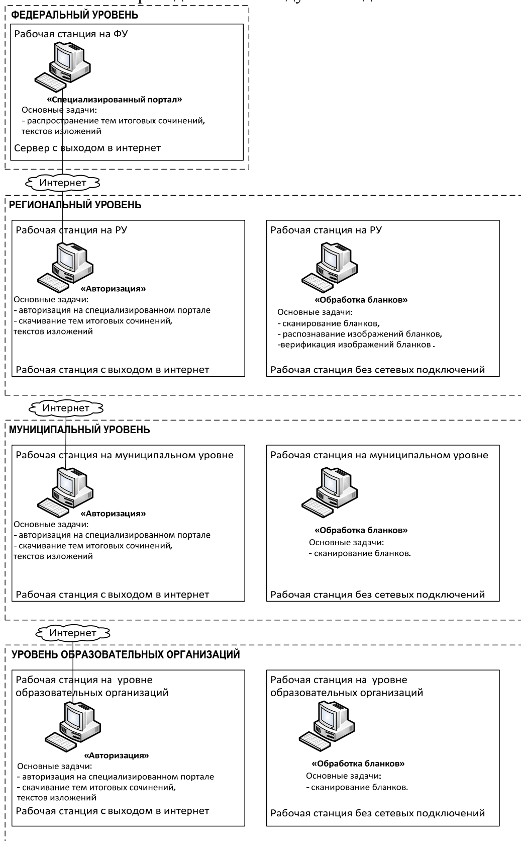
Рисунок 1 – Архитектура и состав ПО
